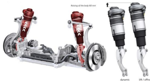
Suspensión neumática adaptativa "S"
